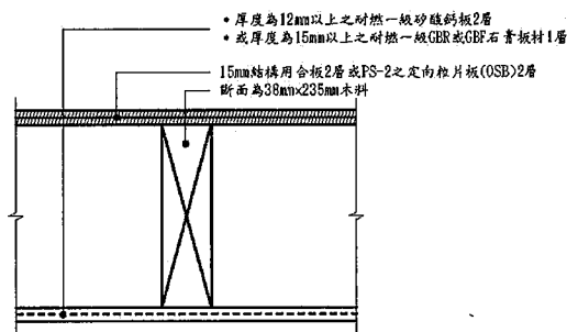
圖9.3-4 半小時防火時效木構造屋頂示意圖
