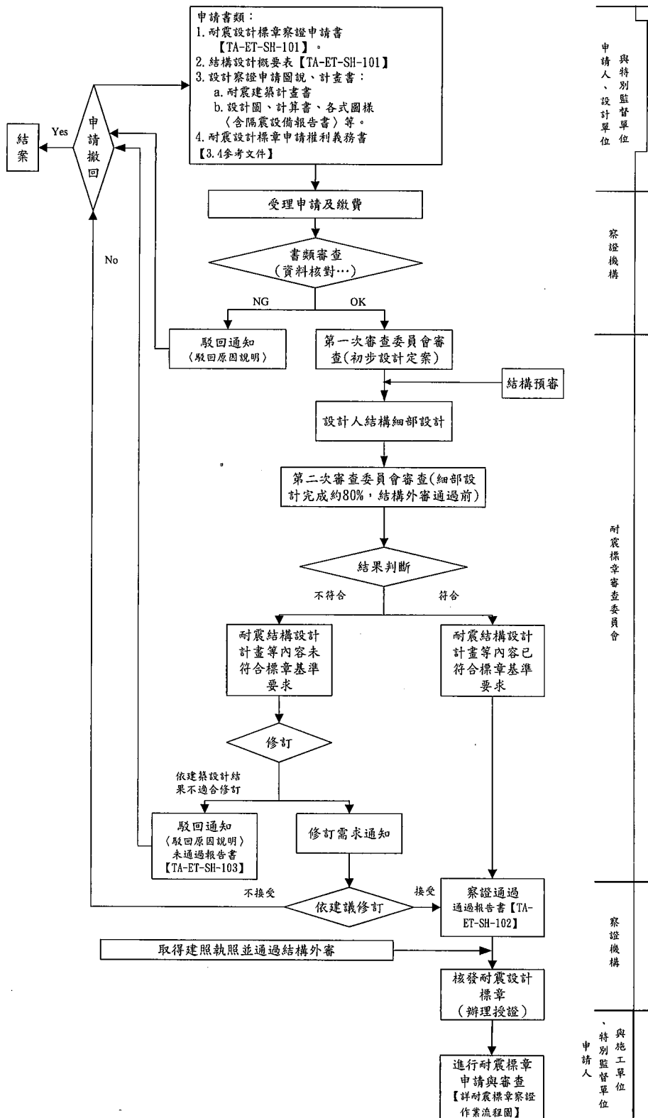
圖一、耐震設計標章審查作業流程圖
