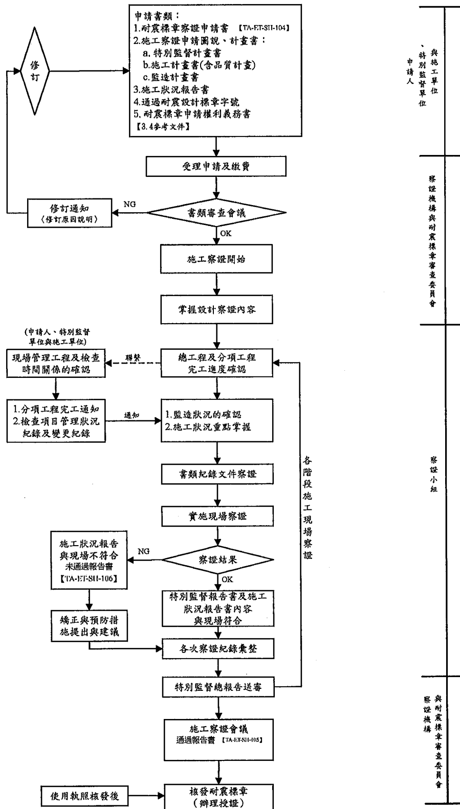
圖二、耐震標章審查作業流程圖
