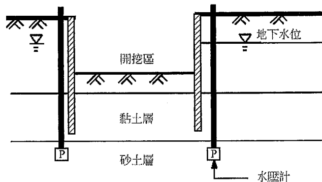
圖 2-12 考慮上舉問題之水壓計佈設剖面示意圖
