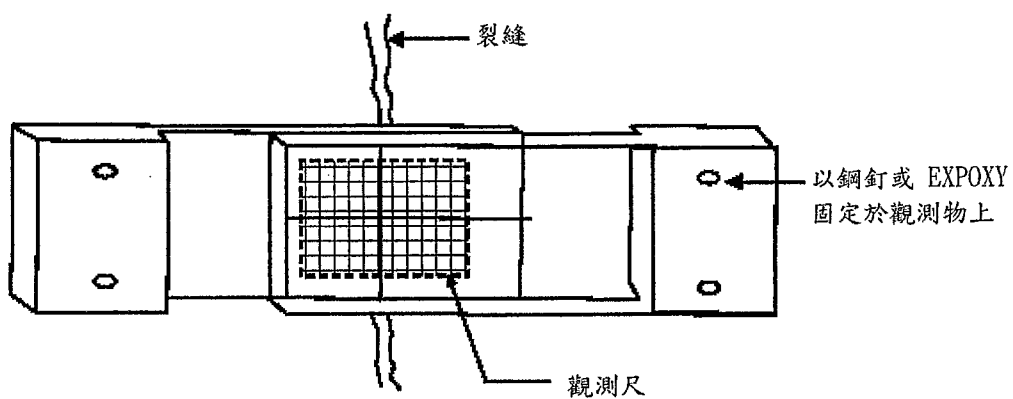
圖 A-15 目視裂縫計示意圖
