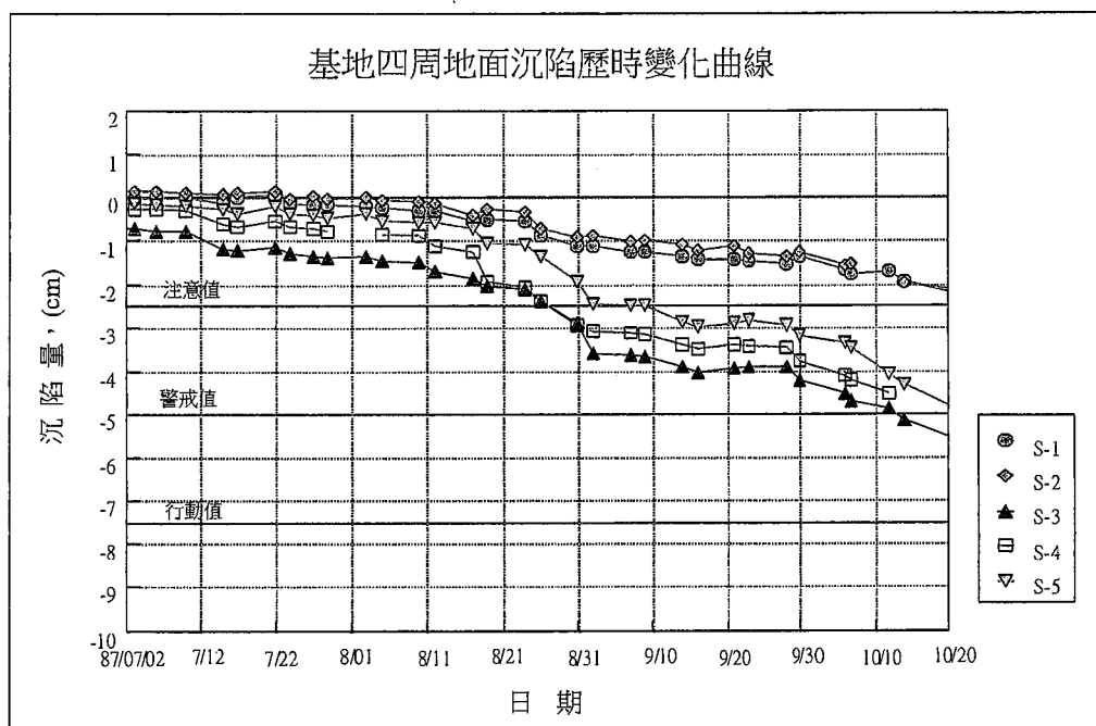
圖 4-7 沉陷觀測點沉陷歷時變化圖例
