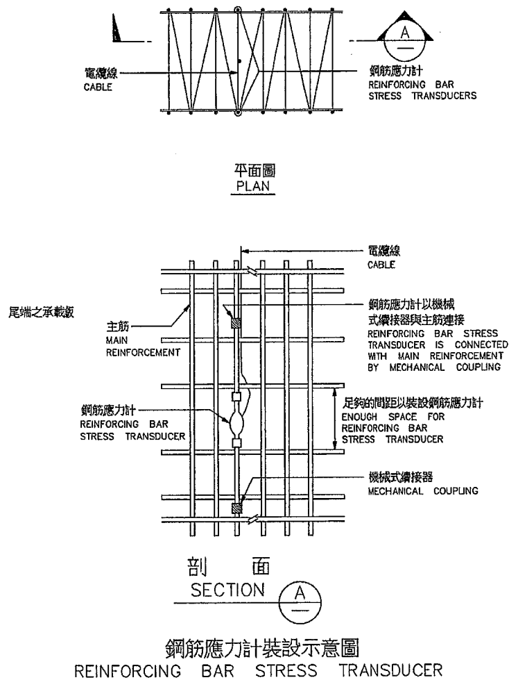
圖 A-4 鋼筋計裝設示意圖
