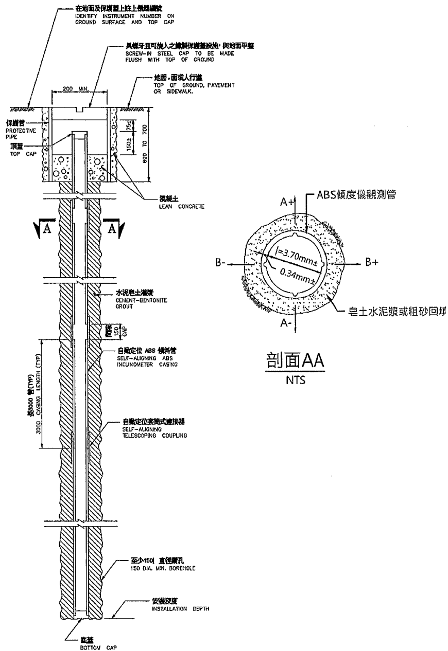
傾度管(土壤中)裝設示意圖 INCLINOMETER CASING IN EARTH
