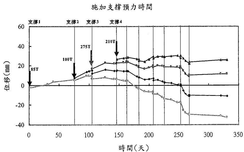
圖 4-2 支撐對應位置之傾度管側向位移歷時變化圖例
