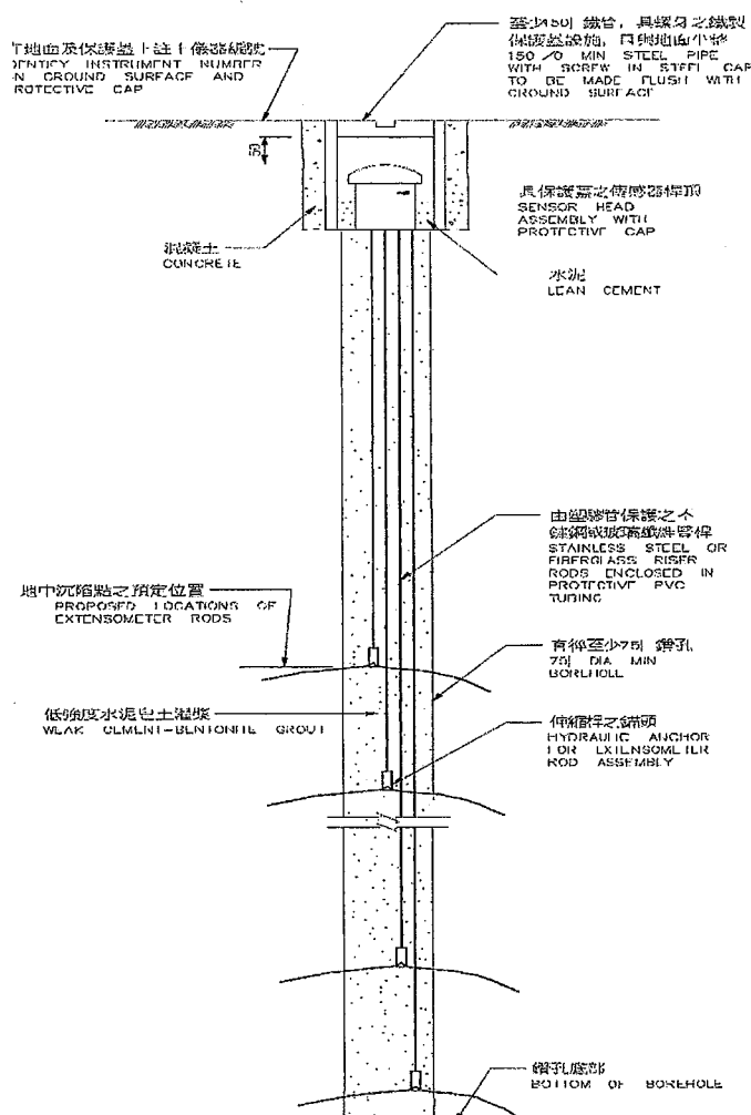
圖 A-9 地中沉陷觀測點示意圖
