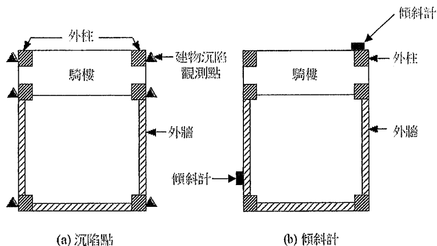
圖 2-15 建物沉陷觀測點及傾斜計配置原則示意
