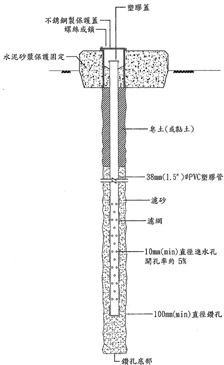
水位觀測井安裝示意圖
