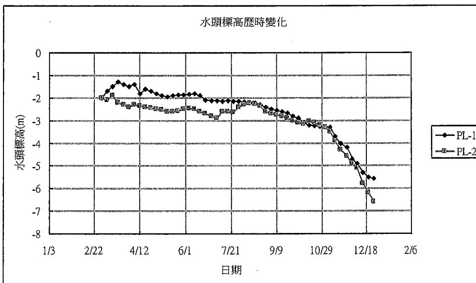
圖 4-6 水位觀測井及水壓計水頭標高歷時變化
