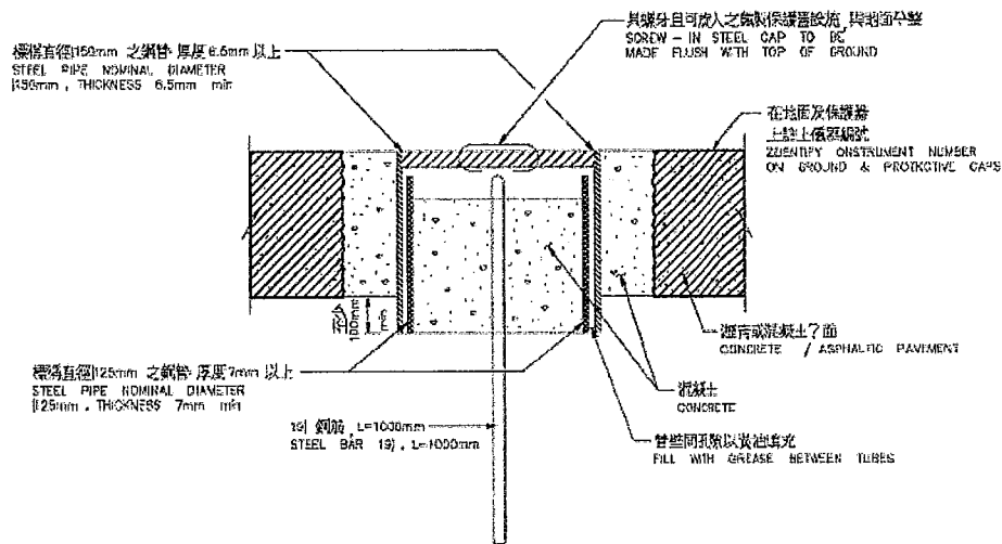
D、沉陷觀測點(淺層部份) 裝設示意圖
